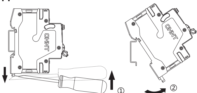
DIN-рейка TH35-7.5
