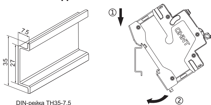
DIN-рейка TH35-7.5
